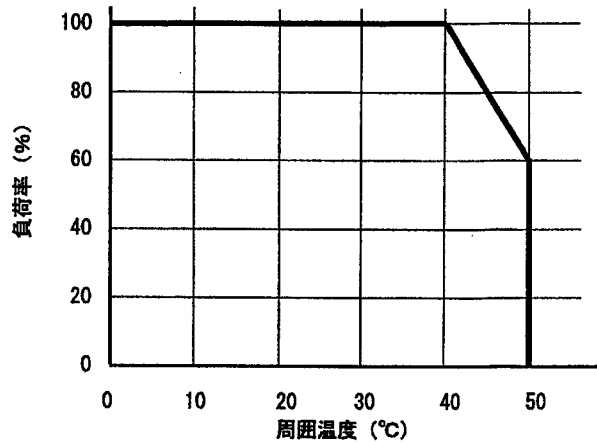
出力電流・電力デレーティング表
