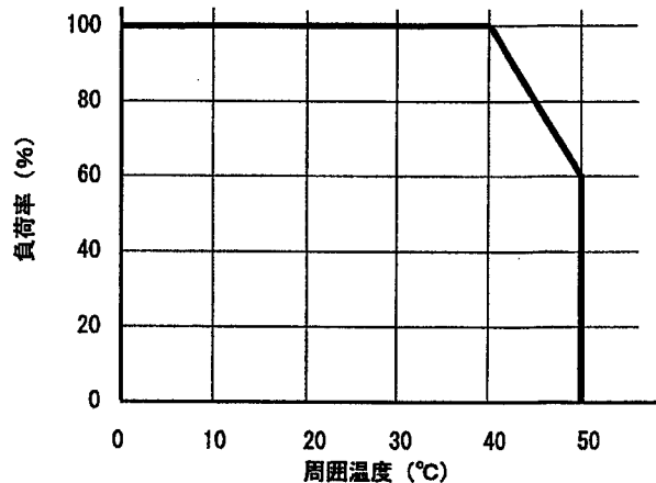
出力電流・電力デレージング表
