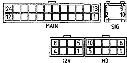
※コネクタピンアサイン詳細図
