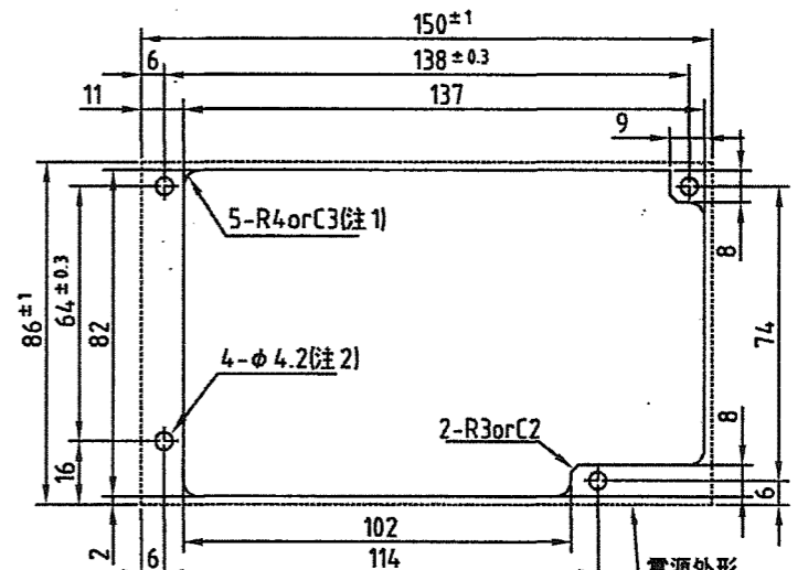
推奨電源取り付け穴加工図
