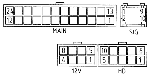
※コネクタピンアサイン詳細図
