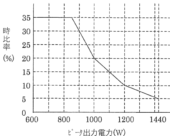
時比率VSピーク出力電力表
