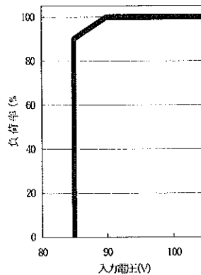
図2. 低入力電圧デレーティング
