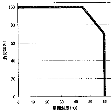
図1. 温度デレーティング
