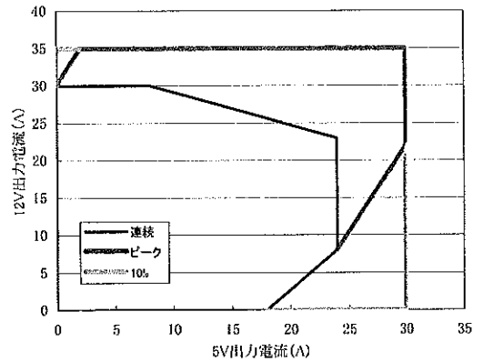
図3. クロスレギュレーション
